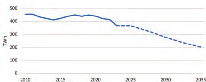
Figure 17. Consommation primaire de gaz fossile à usages énergétiques et non énergétiques, historique (2010-2023) et projetée (2024-2035) (en TWh PCI, périmètre métropole) par «hexagone (avec Corse), hors sources internationales, données historiques corrigées des variations climatiques) – source : SDES (avril 2025), DGEC (dernière version à date du scénario de la Stratégie française énergie-climat)» (Bilan énergétique de la France pour 2023)
