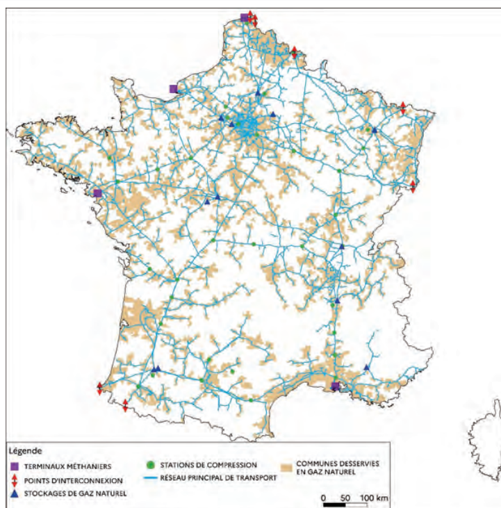
Figure 34. Le réseau gazier français en 2024
