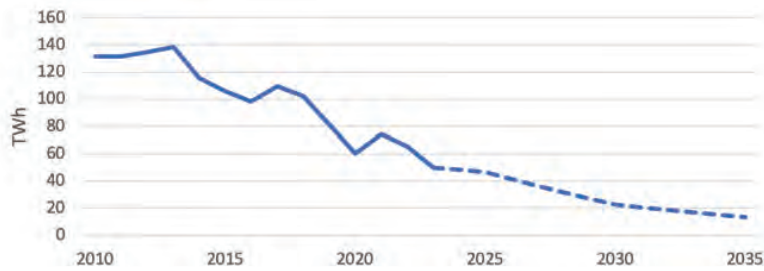
Figure 13. Consommation primaire de charbon à usages énergétiques et non énergétiques, historique (2010-2023) et projetée (2024-2035) (en TWh, périmètre hexagone (avec Corse), hors soutes internationales, données historiques corrigées des variations climatiques) – source : SDES (avril 2025), DGEC (dernière version à date du scénario de la Stratégie française énergie-climat)
